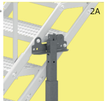
Fixation d'un poteau à l'escalier
