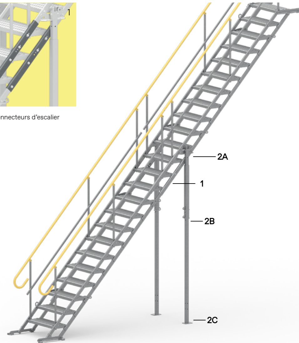
Fixation d'un poteau à l'escalier
